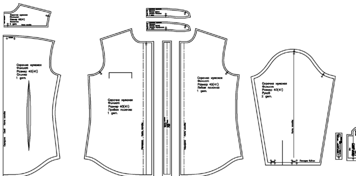
Рис 2. Базовая конструкция мужской сорочки «Финист»
